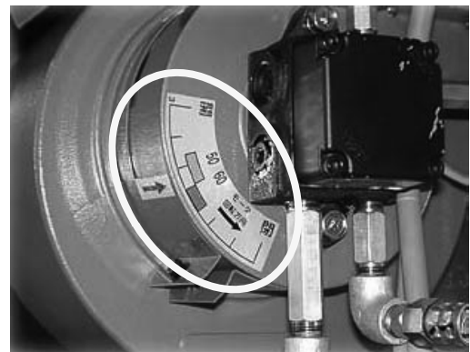
エアシャッターの調整部
