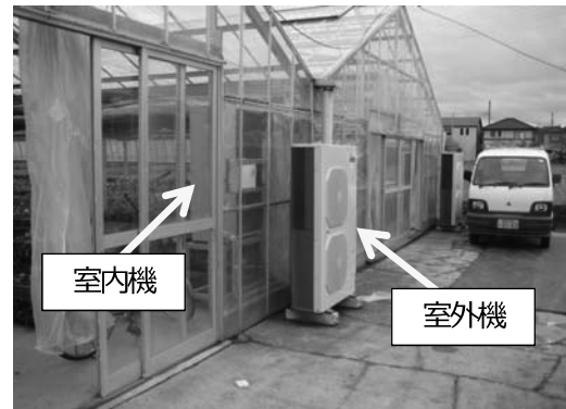
室内機と室外機の適切な設置例
